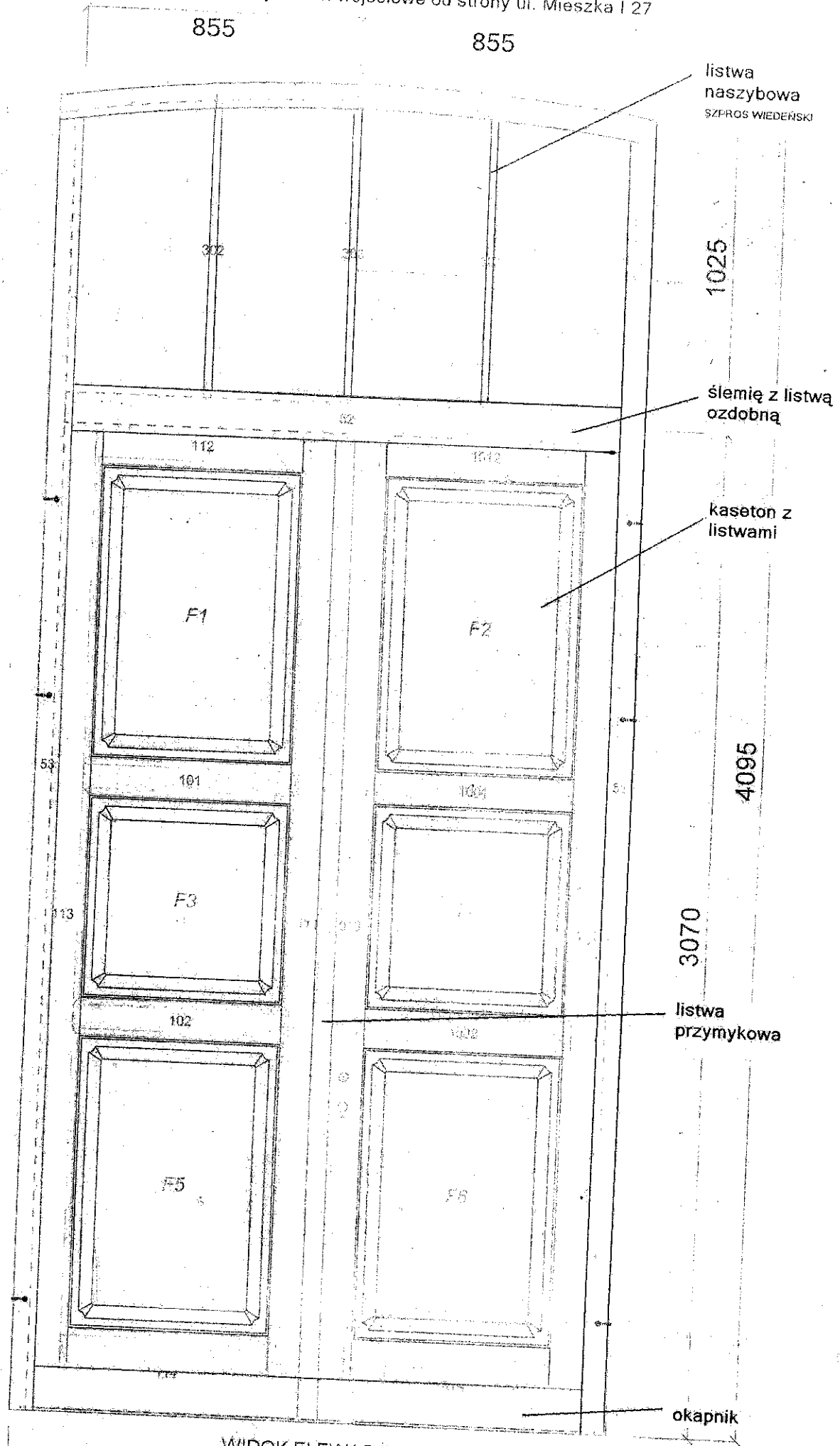
WIDOK ELEWACJI
